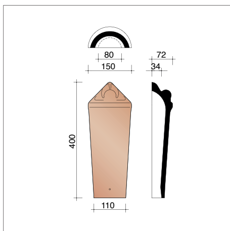
A0003810 Halfronde beginnoordboom
