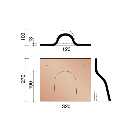
AAR78610 Ventilatiepan zonder rooster - 111 cm 2
