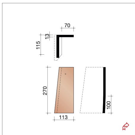
AAR77080 5 stuks/lm Linker gevelpan
