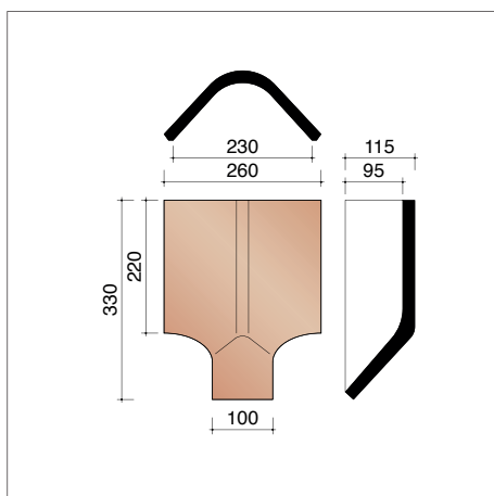
A0005800 Verbindingsstuk tussen 1 vorst 1800 en 2 noordbomen 3700
