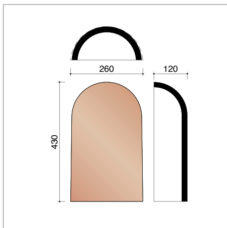
A0001420 Halfronde begin- en eindvorst met kop
