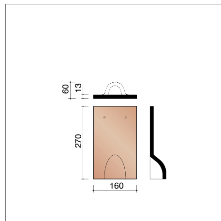
AAR78954 Ventilatiepan 'passe barre' - 34 cm 2
