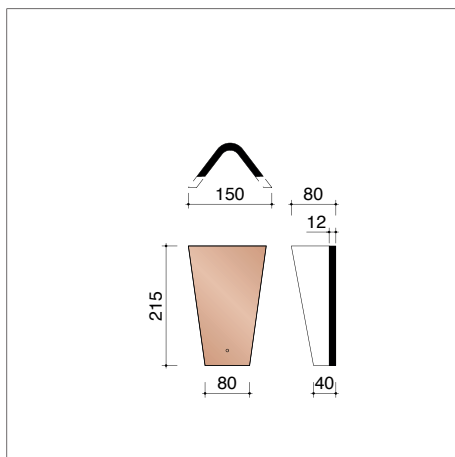
A0003700 10 stuks/lm Kleine hoekige noordboom
