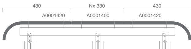
DWARSDOORSNEDE DAK TER HOOGTE VAN VORST 1400 MET QUICK-FIX EXTREME
