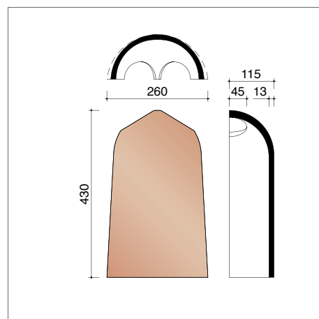
A0005880 Verbindingsstuk tussen 1 vorst 1400 en 2 noordbomen 3700/3800
