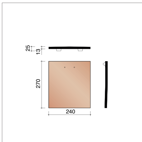
AAR78020 Anderhalve pan
