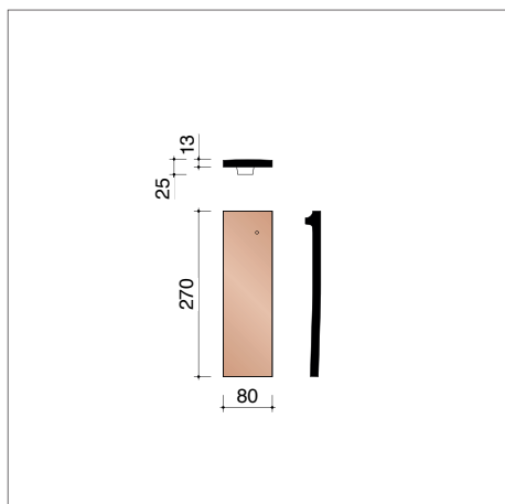
AAR78010 5 stuks/lm Halve pan
