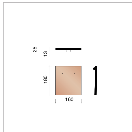
AAR78110 6,3 stuks/lm Korte pan
