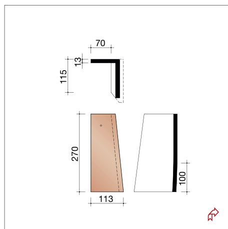
AAR77090 5 stuks/lm Rechter gevelpan
