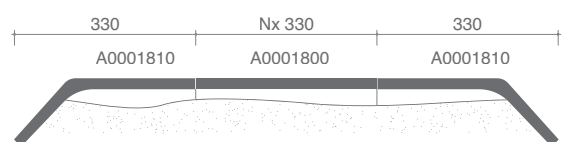
DWARSDOORSNEDE DAK TER HOOGTE VAN VORST 1800 INGEMORTELD
