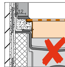
Foute montage (afb. inlegframe)
