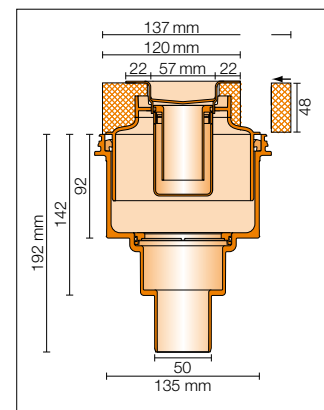
Dwarsdoorsnede
