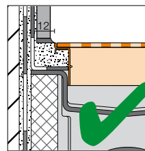
Correcte montage (afb. inlegframe)
