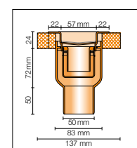
Dwarsdoorsnede middeninbouw
