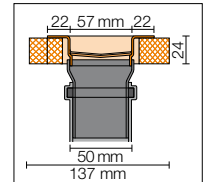
Dwarsdoorsnede middeninbouw
