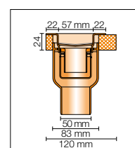
Dwarsdoorsnede wandinbouw
