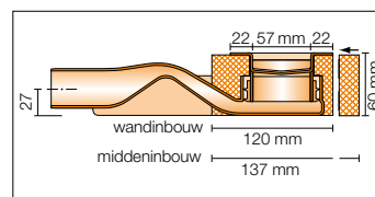
Dwarsdoorsnede
