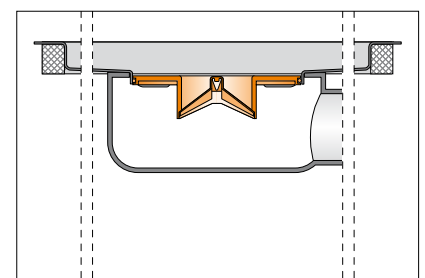
Lengtedoorsnede
