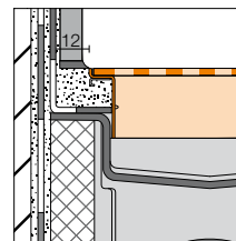
Afb.: inlegrame
