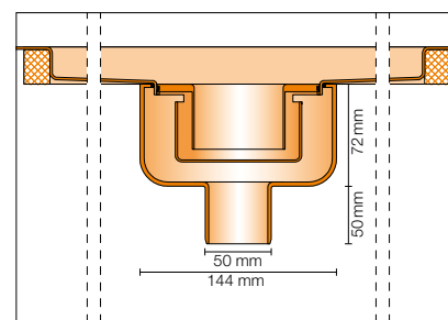
Lengtedoorsnede wand- / middeninbouw
