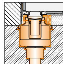
4b Inbouw in wand/plafond
