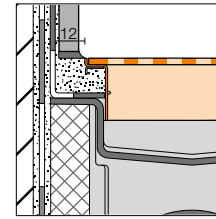
afb. inlegframe
