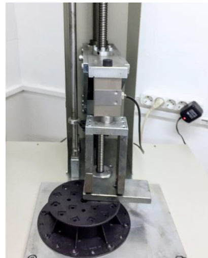
1/4: druklast over een kwart van de tegeldrager
