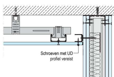
Dragende wandaansluiting met metalen structuur
