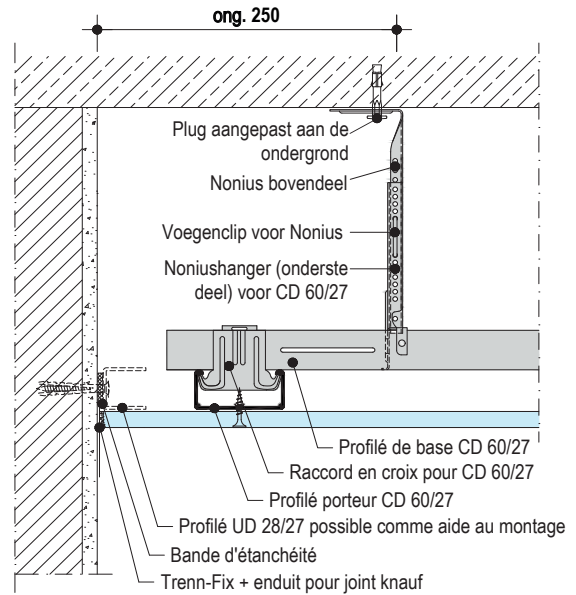
D112 be-D3 Aansluiting met de massieve wand
