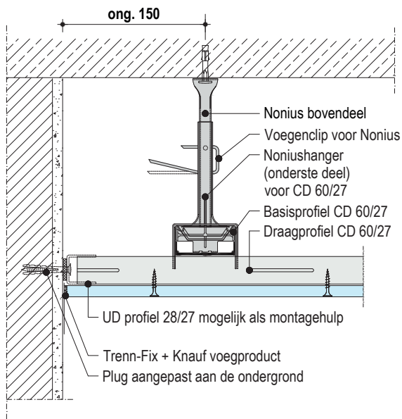
D112 be-A1 Aansluiting met de massieve wand
