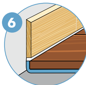
Bevestig de plint enkele millimeters boven het parket en maak een soepele voeg.
