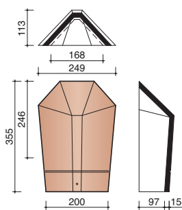
M0001960 Hoekige beginnoordboom Vauban
