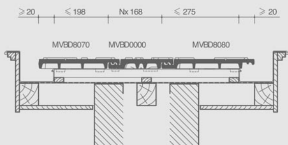
Dwarsdoorsnede dak ter hoogte van anderhalve pan zonder zijsluiting
