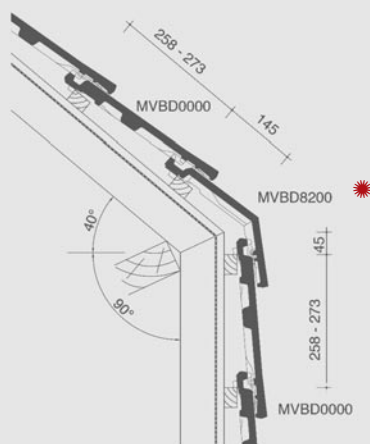
Lengtedoorsnede dak ter hoogte van haakvorst
