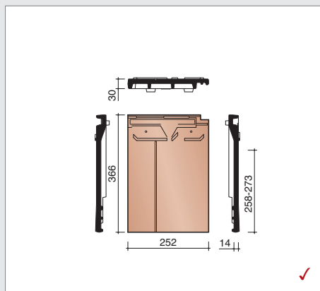
MVBD8070 1,9 stuks/lm Linker anderhalve zijpan zonder sluiting
