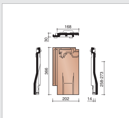
MVBD8640 Ventilatiepan met rooster in kunststof 10 cm 2
