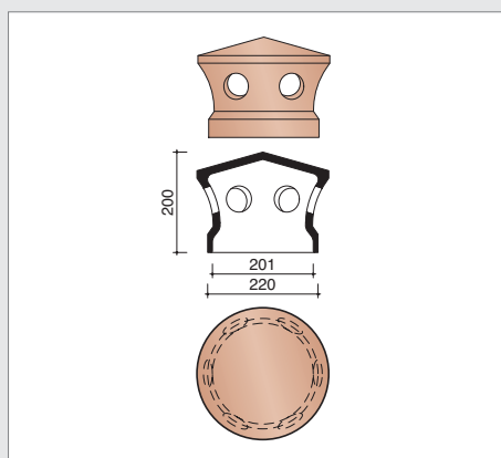
M0008780 Kapje voor kokerpan Ø 150 mm
