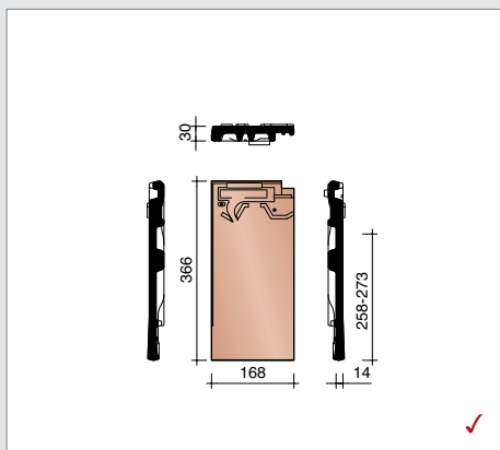
MVBD8045 1,9 stuks/lm Linker zijpan zonder sluiting
