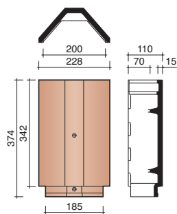
M0002800 3 stuks/lm Hoekige vorst - noordboom Actua
