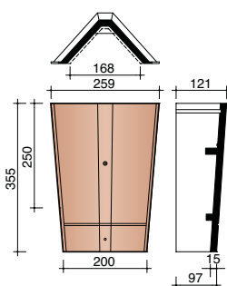
M0001900 4 stuks/lm Hoekige vorst - noordboom Vauban
